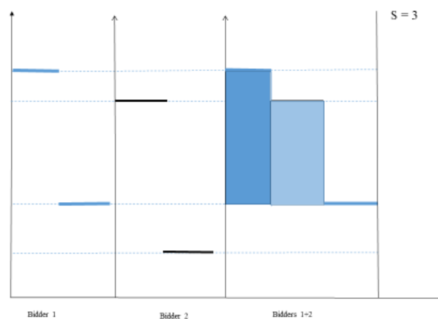
Fig. 2 Asta pay-as-your-bid con N = 2 bidders e K = 3 oggetti identici
