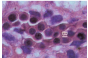
Embryonic globin genes
