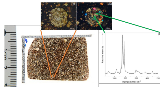
Analisi Raman di condruoli in meteoriti
