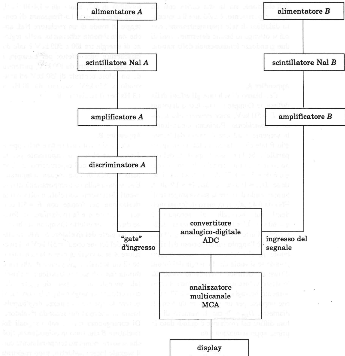
Fig. 8. - Schema della strumentazione elettronica usata nell'esperimento.
