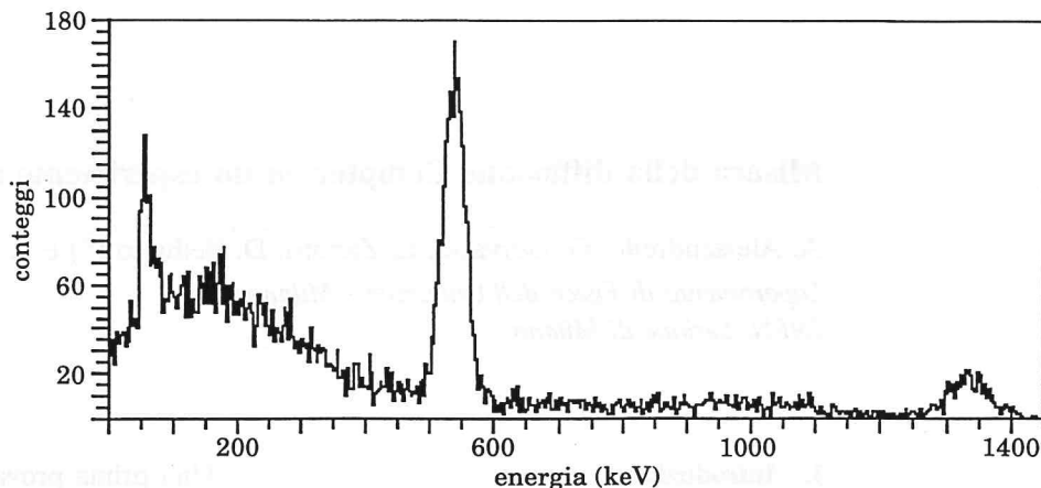
Fig. 1. - Spettro di calibrazione di NaI (2 pollici \times 2 pollici) con sorgente di ^{22}\text{Na} .
