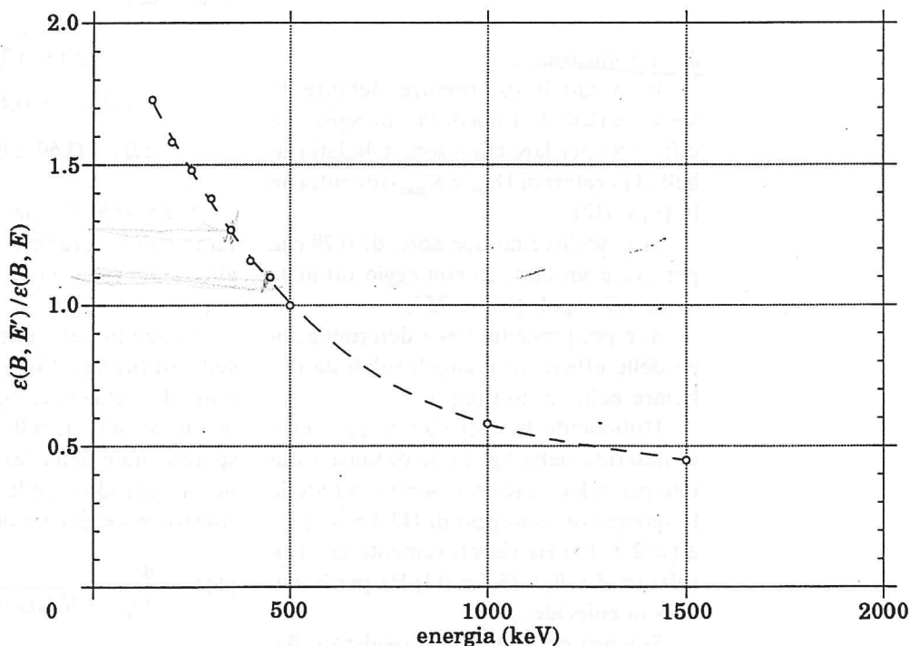
Fig. 5. - Rapporto delle efficienze intrinseche al fotopicco (normalizzate a 511 keV) in funzione dell'energia del fotone incidente.
