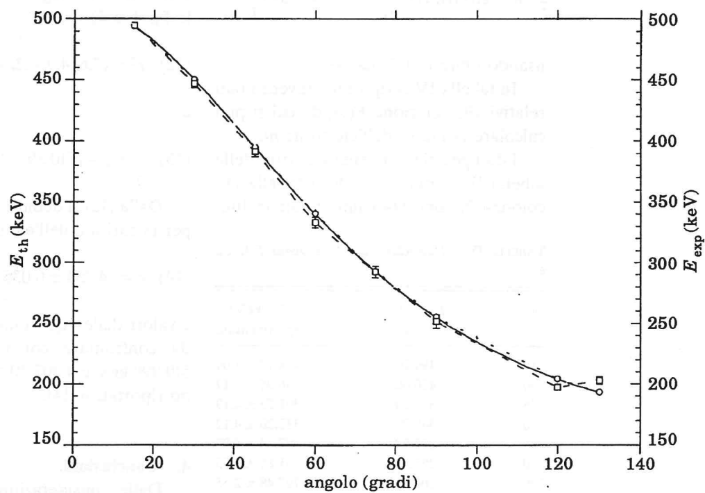
Fig. 7. - Dipendenza dell'energia del fotone diffuso dall'angolo di diffusione: \circ andamento teorico, \square dati sperimentali.
