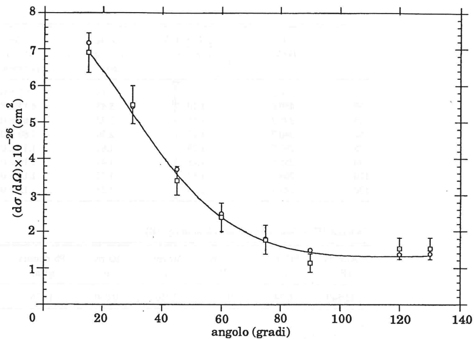
Fig. 6. - Sezione d'urto Compton differenziale d\sigma/d\Omega \cdot 10^{-26} \text{ cm}^2 : \circ teorica, \square sperimentale; la curva continua è l'interpolazione dei dati da cui si ricava il valore di r_e^2 .
