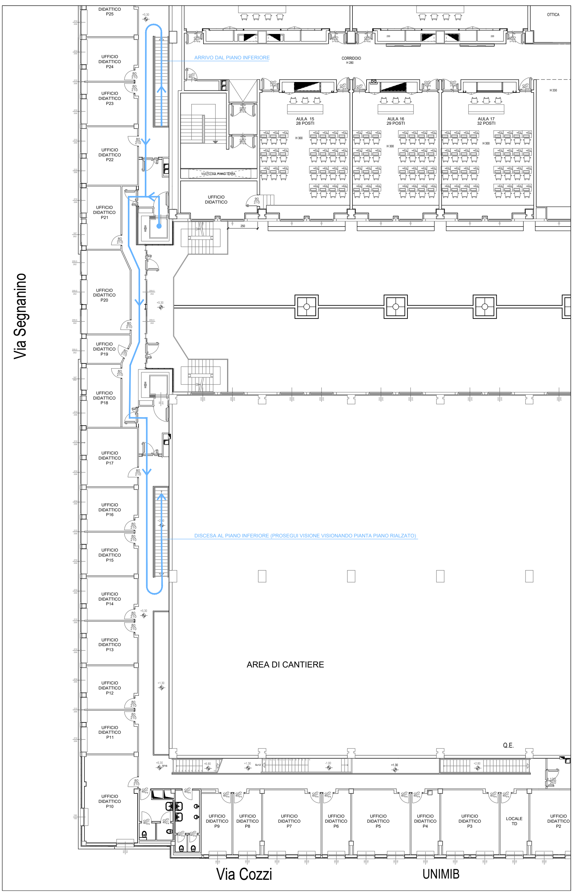
EDIFICIO U9 - STRALCIO PIANTE PIANO PRIMO - PERCORSO ACCESSO LABORATORI DI OTTICA E OPTOMETRIA
