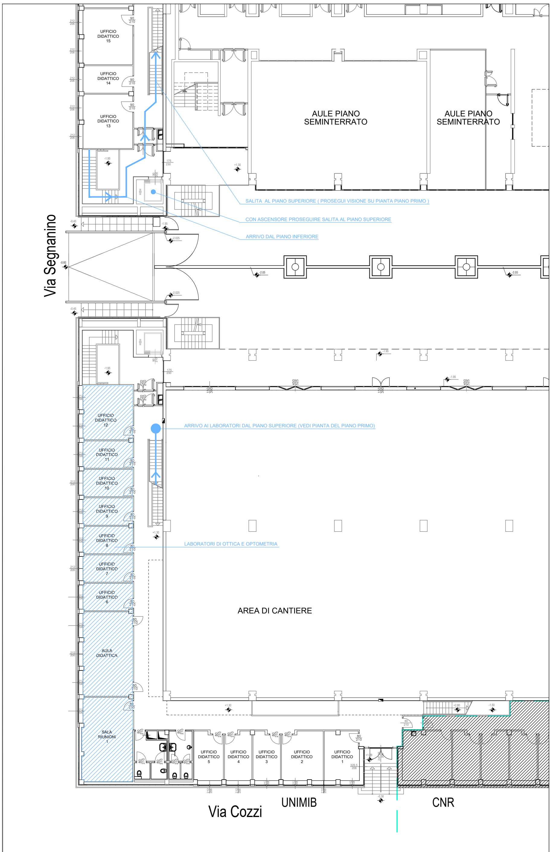
EDIFICIO U9 - STRALCIO PIANTA PIANO RIALZATO - PERCORSO ACCESSO LABORATORI DI OTTICA E OPTOMETRIA
